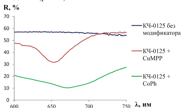
Рис. 2. Сравнительные спектры отражения водоразбавляемых композиций.
