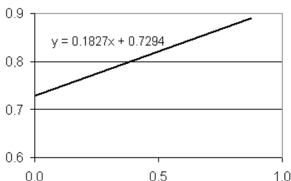
Рис 3. Зависимость \eta_{\text{уд}}/C от \eta_{\text{уд}} (раствор хлорированного поливинилхлорида в бутилацетате).
