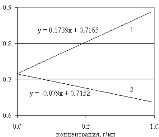
Рис 2. Зависимость \eta_{\text{уд}}/C (1) и \ln \eta_{\text{отн}}/C (2) от концентрации раствора (раствор хлорированного поливинилхлорида в бутилацетате).
