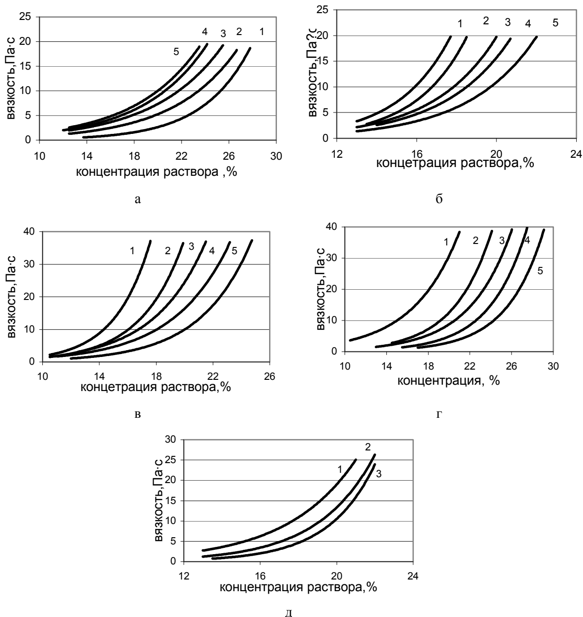
Рис. 4. Зависимость динамической вязкости от концентрации растворов: а – ПХВ+СКН-26-1А; б – ПХВ+БНКС-28АМН; в – ПХВ+ Desmocoll 400; г – САН+ Desmocoll 400; д – ПХВ+ Наирит ДП (содержание эластомера 1 – 0 масс. %; 2 – масс. 10%; 3 – масс. 20%; 4 – масс. 30%; 5 – масс. 50%).
