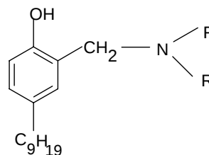
Рис. 1. N -(2-гидрокси-5-нонилбензил)-диалкиламин (НБАА); R = C_nH_{2n+1}
