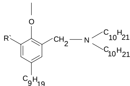
Рис. 3. Анион НБДА- R' ( R^- ), где R' = OH, NO_2, F, Cl, Br, I .
