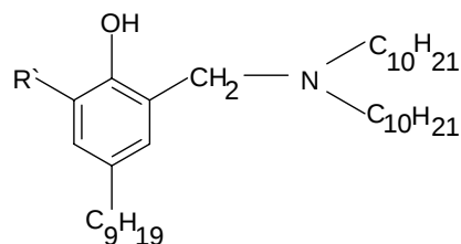
Рис. 2. Замещенный в о -положении N -(2-гидрокси-5-нонилбензил)-дидециламин, НБДА- R' ( HR ), где R' = OH, NO_2, F, Cl, Br, I .
