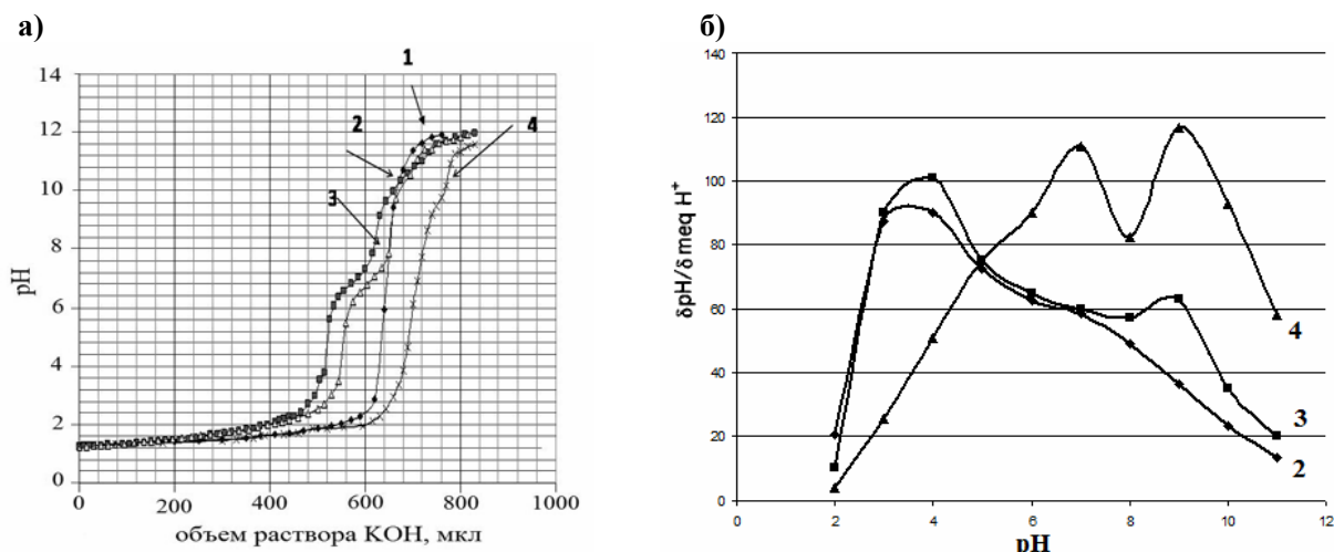
Рис. 3. Быстрое потенциметрическое титрование целых клеток в среде 0.001 М KCl и 0.1 М HCl раствором 1 М KOH: 1 – без клеток (контроль); 2 – M. quaylei MT; 3 – M. quaylei SM+; 4 – S. maltophilia . а) Кривые титрования; б) дифференциальные кривые титрования.
