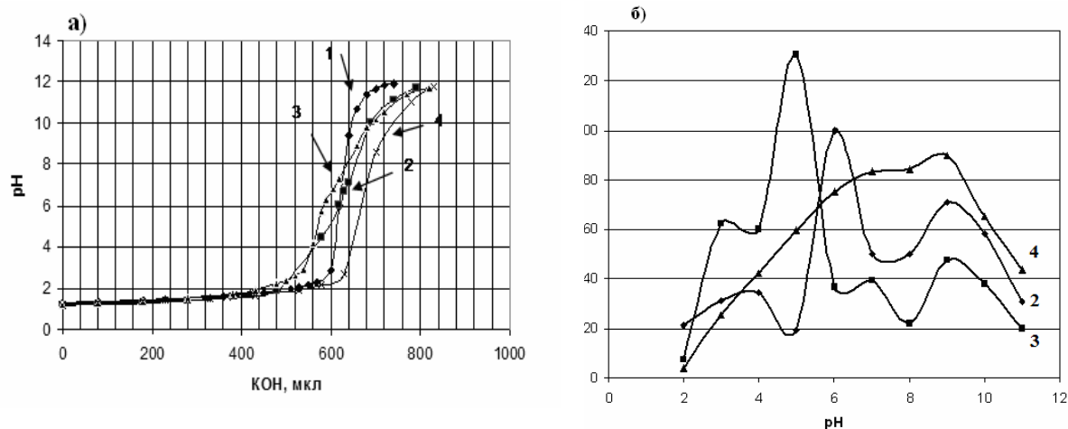
Рис. 4. Быстрое потенциметрическое титрование целых клеток, выращенных в присутствии ОК ( 5.0 \cdot 10^{-5} М), в среде 0.001 М KCl и 0.1 М HCl раствором 1 М KOH: 1 – без клеток (контроль); 2 – M. quaylei MT; 3 – M. quaylei SM+; 4 – S. maltophilia .
