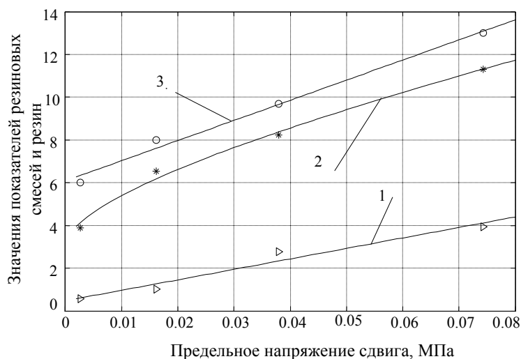
Рис. 4. Зависимости характеристик резиновых смесей и резин от предельного напряжения сдвига в модельных дисперсиях технического углерода УМ76 в ДБФ:
