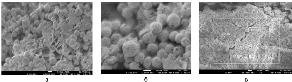
Рис. 5. Фотографии СЭМ композита \eta -TiO 2 /Y 2 O 3 с разрешением \times 50000 (а), \times 100000 (б), \times 450 (в).
