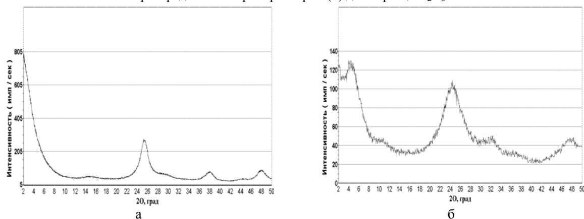
Рис. 3. Дифрактограммы образца 1 с анатазом (а) и образца 2 с \eta\text{-TiO}_2 (б).
