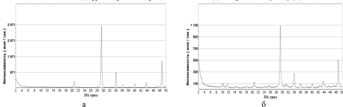
Рис. 4. Дифрактограммы композита анатаз/ \text{Y}_2\text{O}_3 (а) и \eta\text{-TiO}_2/\text{Y}_2\text{O}_3 (б).
