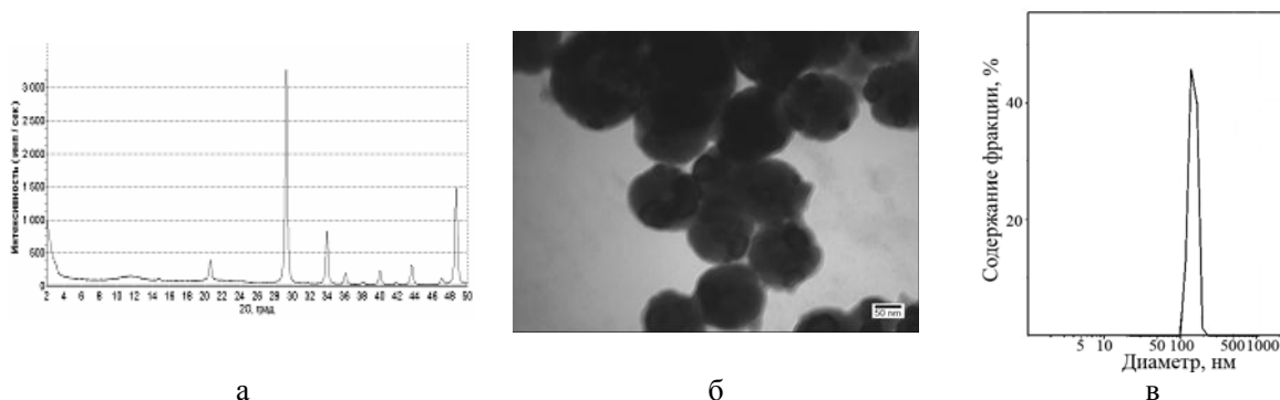
Рис. 1. Дифрактограмма (а), фотография ПЭМ (б) и распределение частиц по размерам (в) образца \text{Y}_2\text{O}_3 .
