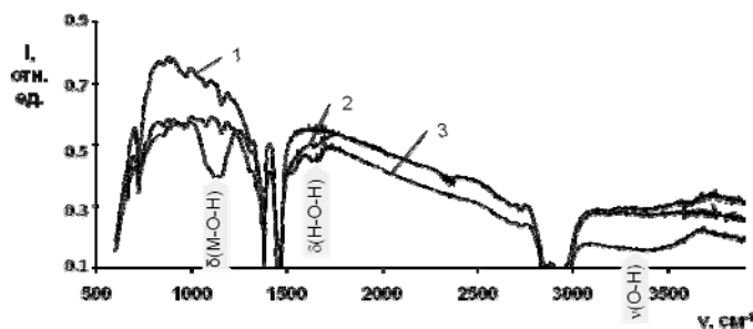
Рис. 8. ИК-спектры образцов: 1 – чистый \text{Y}_2\text{O}_3 ; 2 – микросферы \text{Y}_2\text{O}_3 , модифицированные наночастицами \eta\text{-TiO}_2 в щелочной среде; 3 – микросферы \text{Y}_2\text{O}_3 , модифицированные титаноксидными наночастицами путём диспергирования оксида иттрия в кислотном гидрозоле, полученном 180-секундным гидролизом сульфата титанила.
