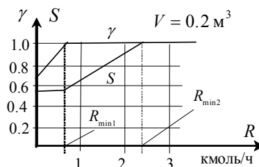
Рис. 7. Зависимость конверсии \gamma и селективности S от величины потока рецикла.
