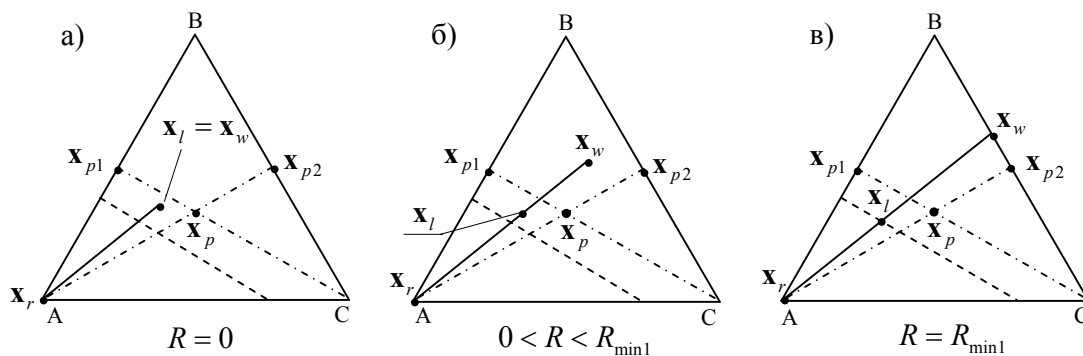
Рис. 4. Эволюция стационарных состояний в зависимости от потока рецикла. (прямая сплошная линия – линия материального баланса ректификационной колонны; пунктирная линия – линия изопроизводительности, соответствующая полной конверсии)
