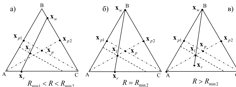
Рис. 5. Эволюция стационарных состояний системы в зависимости от потока рецикла. (прямая сплошная линия – линия материального баланса ректификационной колонны; пунктирная линия – линия изопроизводительности, соответствующая полной конверсии).
