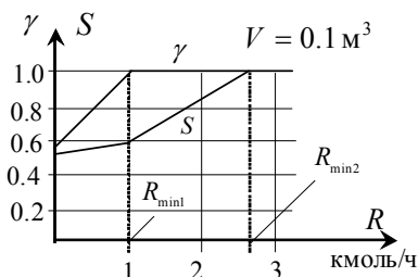
Рис. 6. Зависимость конверсии \gamma и селективности S от величины потока рецикла.
