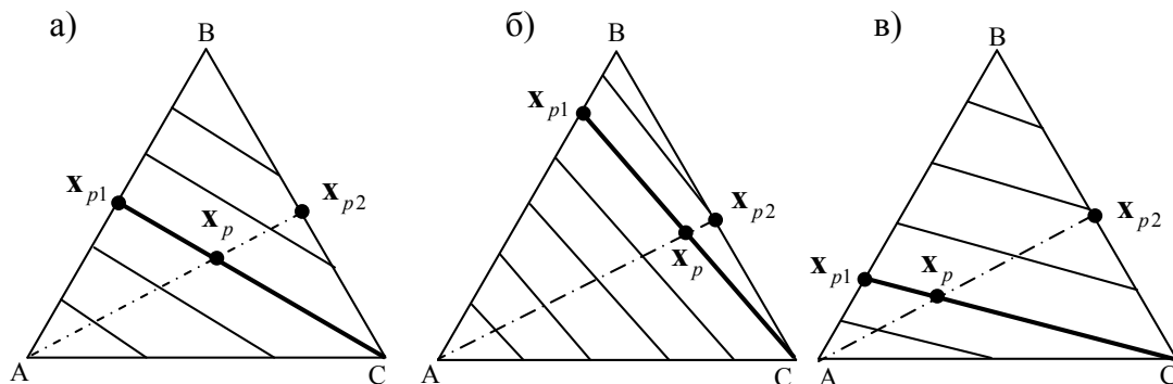
Рис. 2. Расположение линий изоскоростей расхождения реагента А в зависимости от соотношения констант скоростей реакций: а) k_1^+ = k_1^- ; б) k_1^+ > k_1^- ; в) k_1^+ < k_1^- . (жирная прямая линия – линия нулевой скорости превращения реагента А; штрихпунктирная – линия нулевой скорости образования продукта С).
