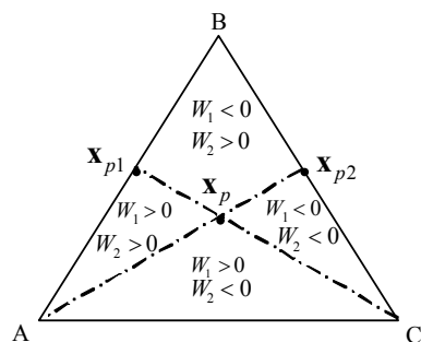
Рис. 3. Линии нулевых изоскоростей по реагенту А и продукту С.
