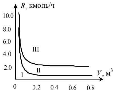
Рис. 8. Зависимость величин потока рецикла от объема реактора. (области: I – \gamma < 100\% , S < 100\% ; II – \gamma = 100\% , S < 100\% ; III – \gamma = 100\% , S = 100\% ).
