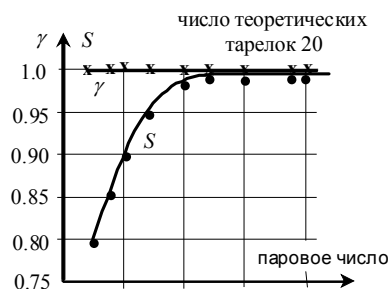
Рис. 11. Зависимость конверсии и селективности от величины парового числа.
