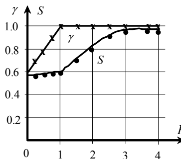
Рис. 9. Зависимость конверсии и селективности от рецикла при конечной эффективности по разделению.
