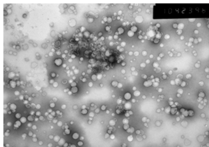
Рис. 3. Микрофотография липосом липидного состава ДПФХ-ХС (7:3) с карнозином, полученных методом активной загрузки (увеличение 10 000×).
