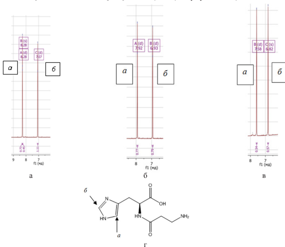
Рис. 1. Фрагменты ^1\text{H} -ЯМР-спектров карнозина в водных растворах при различных pH: а) 6.3; б) 7.1; в) 8.2 в области сигналов протонов a и б имидазольного кольца карнозина (г).
