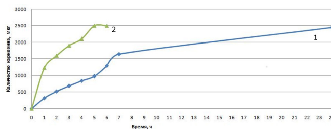
Рис. 4. Кинетика высвобождения карнозина из липосом с липидным составом ДПФХ-ХС (7:3) (1) и диффузия карнозина из контрольного раствора, C_{\text{карнозина}} = 2.5 \text{ мг/мл} (2), определенные с помощью ячейки Франца.
