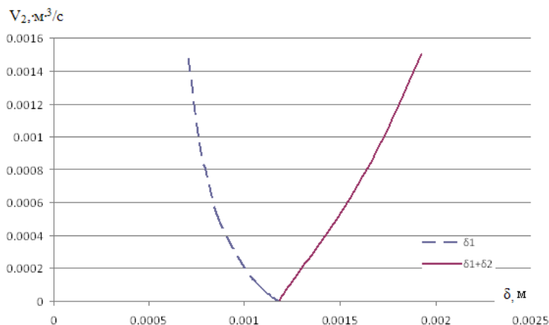
Рис. 3. Зависимость толщин пленок от расхода внешней пленки (при небольшой скорости газа его массовый расход 20 г/с, расход жидкости первой пленки постоянный и составляет 0.5 л/с).
