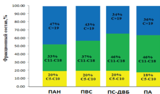
Рис. 3. Фракционный состав продуктов FTS, полученных в системе Fe-парафин-полимер при температуре 320°C.
