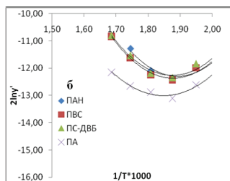
Рис. 5. Зависимости функции \ln Y от 1/T : а) механизм I; б) механизм II.
