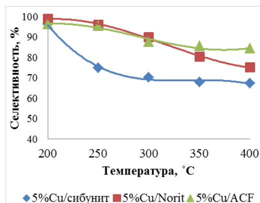
Рис. 2. Зависимость селективности по ацетальдегиду в присутствии медных катализаторов на основе различных углеродных материалов от температуры.
