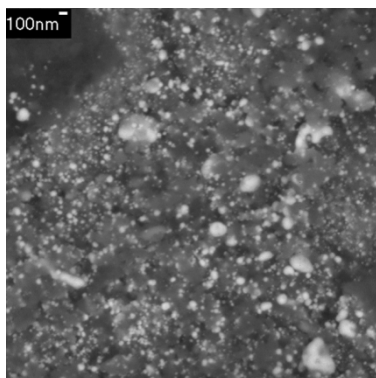
Рис. 5. Изображение SEM поверхности катализатора 5%Cu/сибунит.
