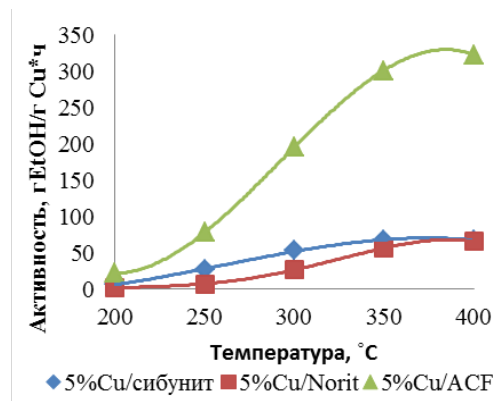
Рис. 3. Зависимость активности медных катализаторов на основе различных углеродных материалов от температуры.
