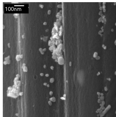
Рис. 6. Изображение SEM поверхности катализатора 5%Cu/Norit.
