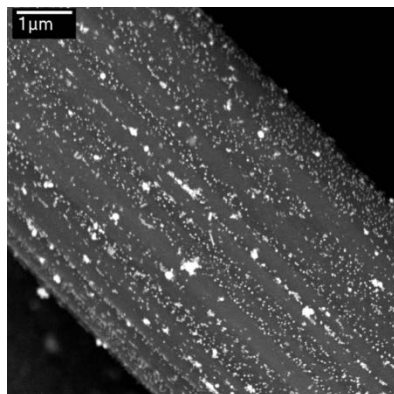
Рис. 7. Изображение SEM поверхности катализатора 5%Cu/ACF при разном увеличении.
