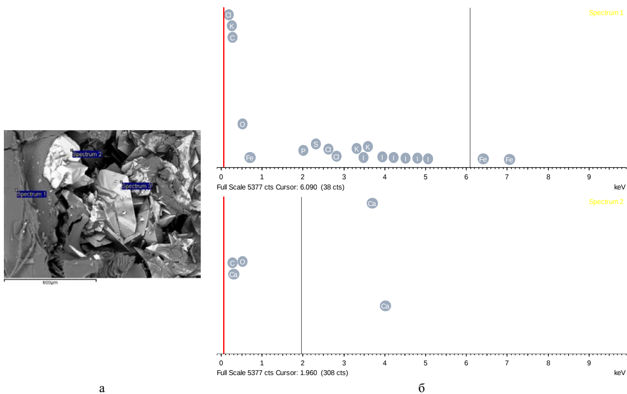
Рис. 3. Микрофотография (а) и энергодисперсионные спектры (б) различных участков мочевого камня 23.
