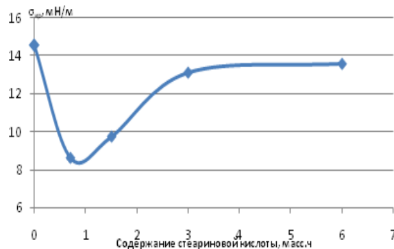
Рис. 4. Зависимость критического поверхностного натяжения образцов каучука ДССК 2560 от содержания стеариновой кислоты.
