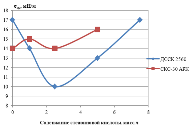
Рис. 5. Зависимость критического поверхностного натяжения образцов резин от содержания стеариновой кислоты.
