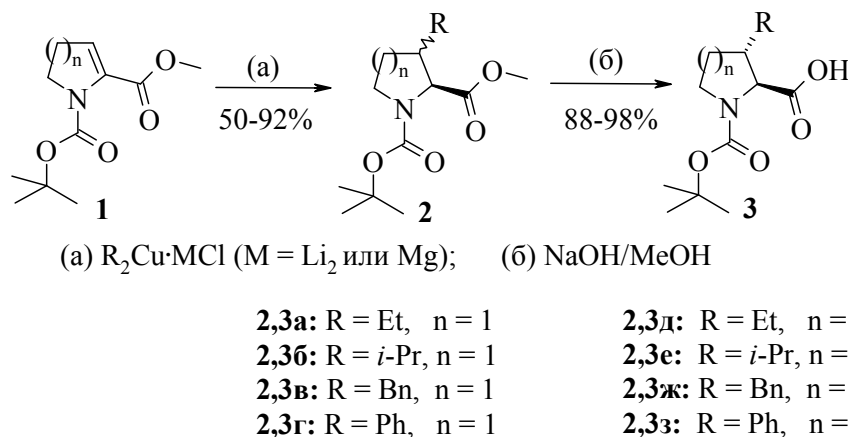
Схема 1. 1,4-Присоединение купратных реагентов, полученных из \text{CuCl} (I) и соответствующих металлоорганических соединений.
