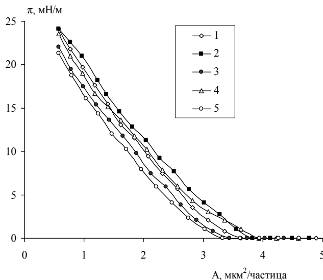
Рис. 2. Изотермы сжатия 2D пленок, сформированных из полистирольных микросфер образца 2 (содержание на поверхности кроме сульфогрупп — фрагментов молекул инициатора, персульфата натрия, сульфогруппы ионогенного сомономер, стиролсульфоната натрия) при различной концентрации (моль/л) сульфата аммония в субфазе: 1 — 0; 2 — 0.1; 3 — 0.2; 4 — 0.3; 5 — 0.4. T = 293\text{ K} .
