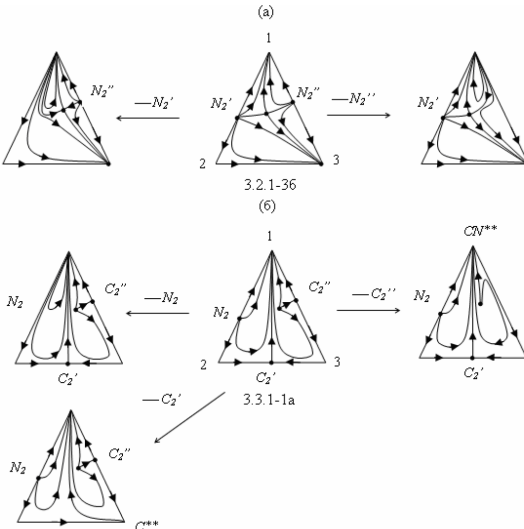
Рис. 7. Примеры «жестких» структур, когда ни один из бинарных азеотропов не может исчезнуть раньше тройного: а) 3.2.1-36; б) 3.3.1-1а.
