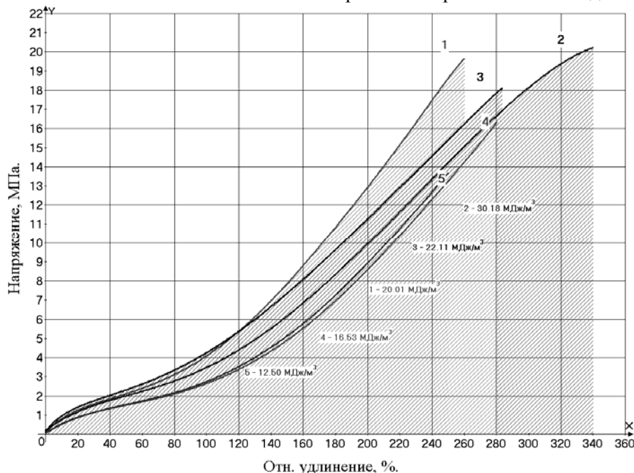
Рис. 1. Удельная работа деформации на разрушение вулканизатов для образцов 1 – 5 (1 – исх. ТУ, 2 – Мод. ТУ, 3 – Мод. ТУ с силианом, 4 – Канальный ТУ, 5 – Канальный ТУ с силианом).
